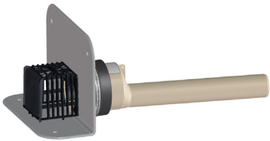
Bild 1 Attikaablauf HL68H.0/DN, HL68P.0/DN, HL68F.0/DN mit Laubfangkorb HL068.1E oder Laubfangkorb zur Notentwässerung HL068.1Safe
